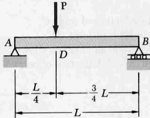
Fig. P10.114
